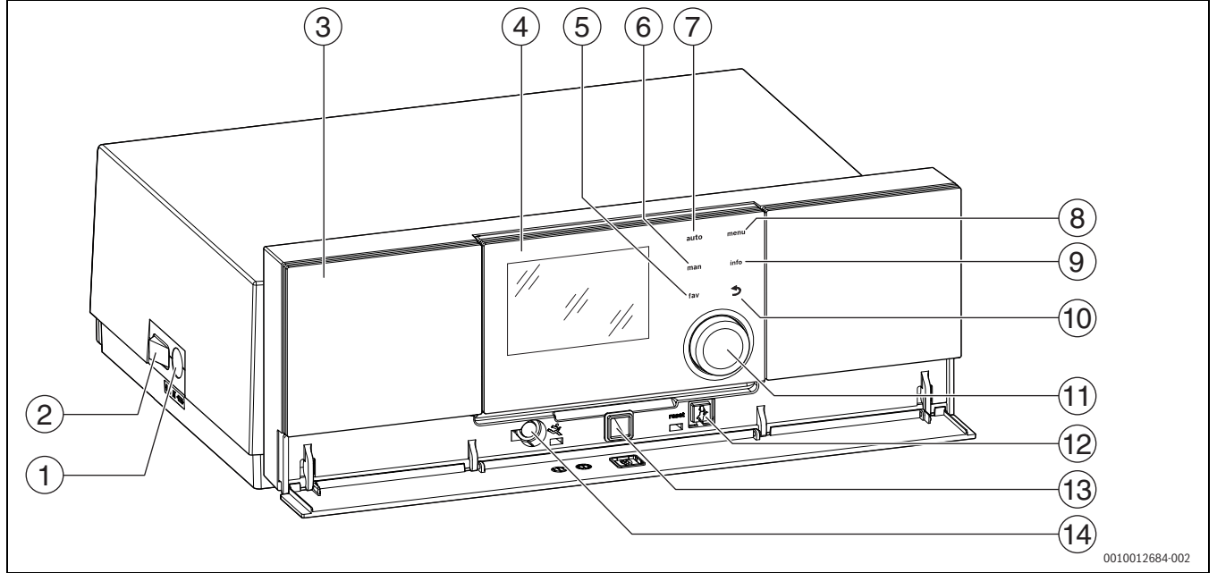
Res. 2 Logamatic RC310 kontrol paneli donanımlı MC110 kumanda paneli – Kumanda elemanları
