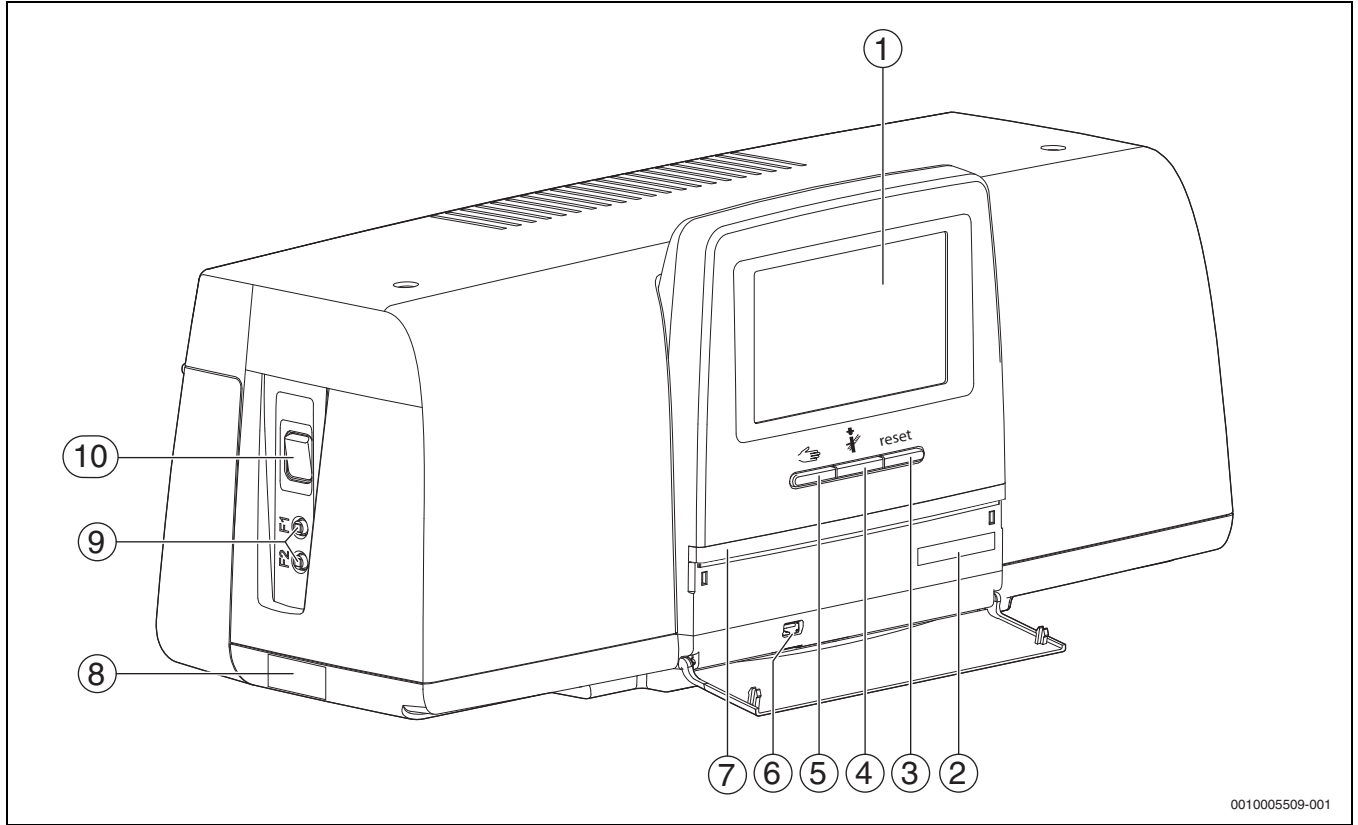
Res. 7 Kumanda elemanları
