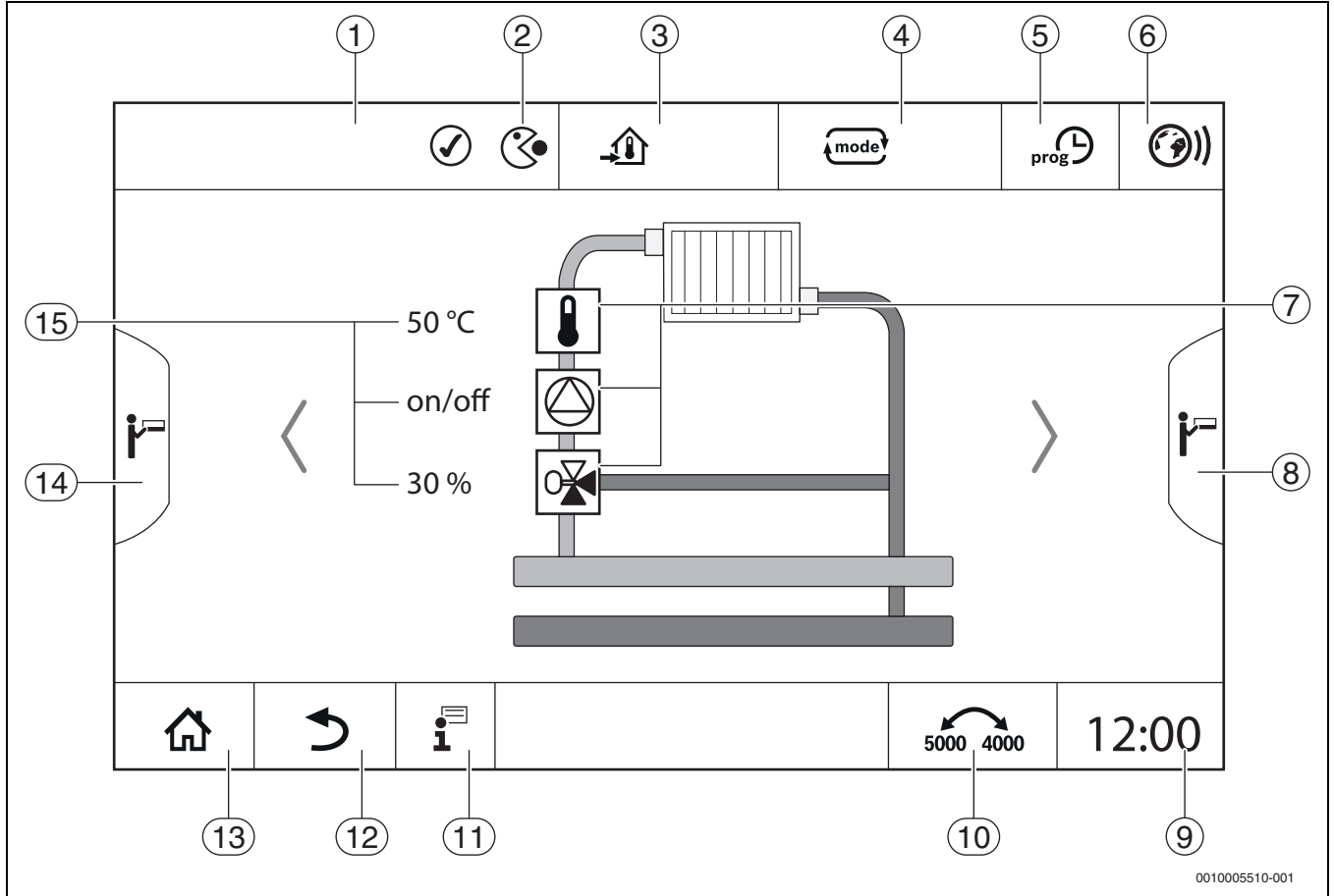
Res. 9 Kumanda ve gösterge elemanları
