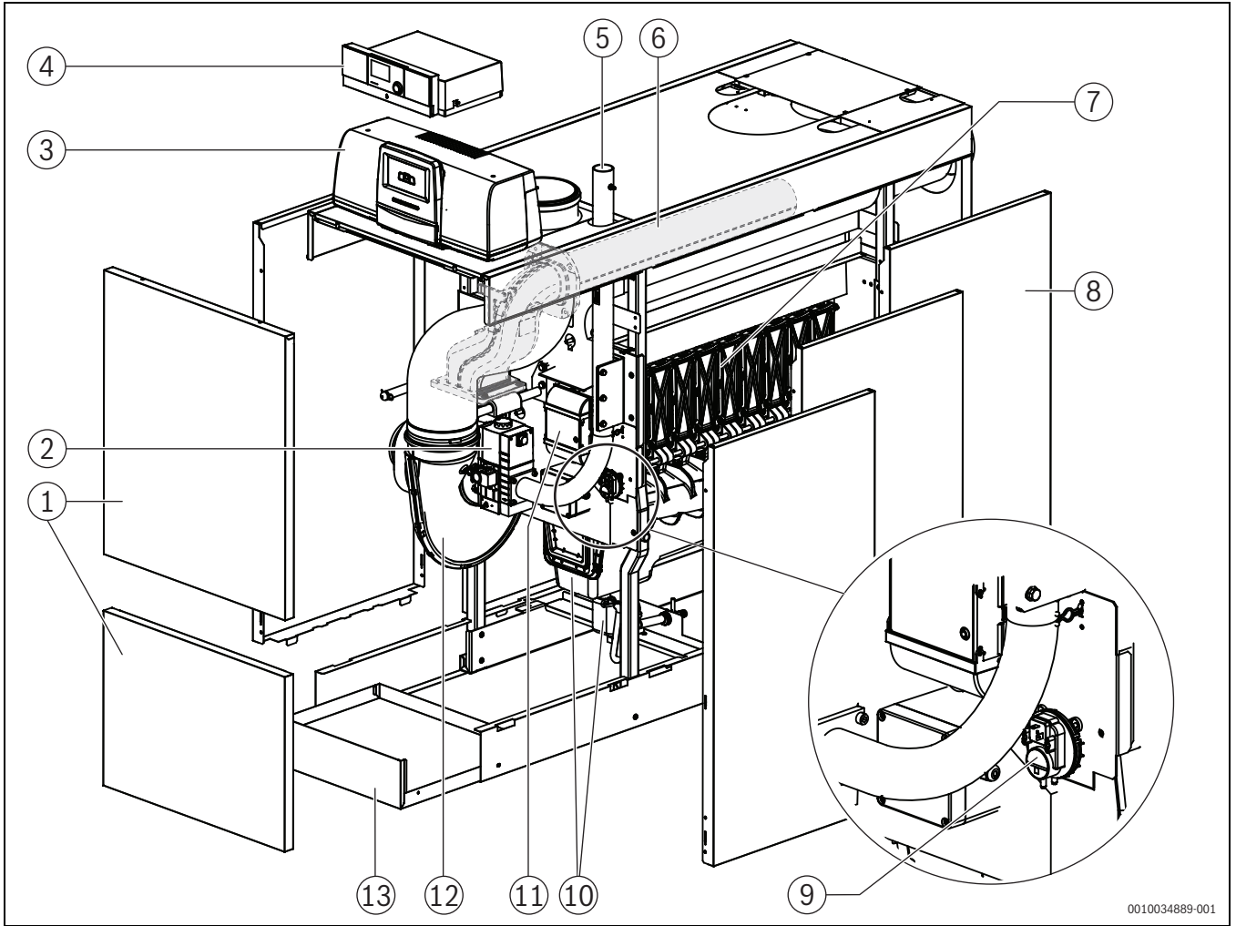
Res. 1 Logano plus KB472, 350...500 kW ana yapı parçaları (gösterilen: sağ model; temizlik kapağı ve gidiş ve dönüş hattı sağ taraftadır)
